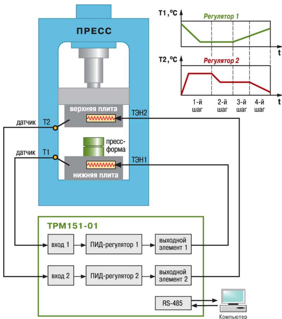
Рисунок 4.2 – Использование 2-канального регулятора TPM151 01й модификации для поддержания температуры в заданных диапазонах при прессовании изделий
