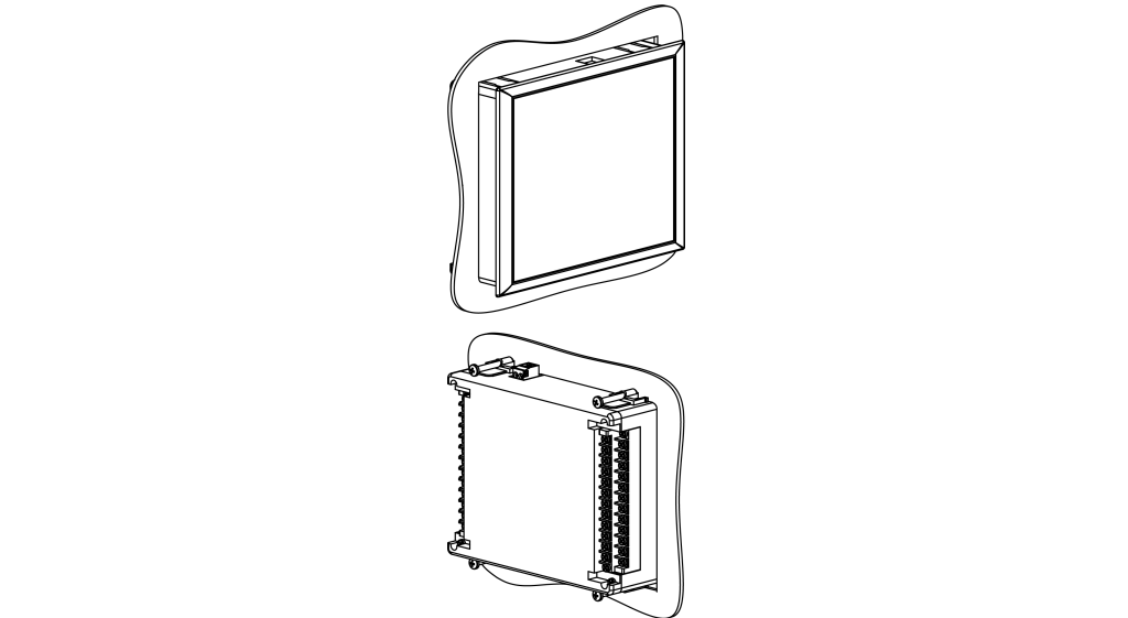
Рисунок 4 – Монтаж прибора щитового крепления
