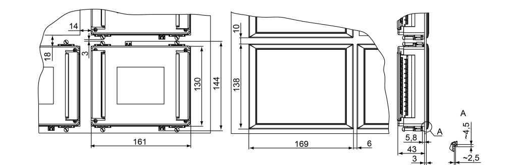
Рисунок 6 – Прибор в корпусе Щ7, установленный в щит толщиной 3 мм
