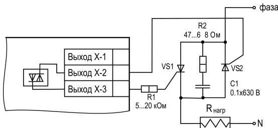
Рисунок 16 – Схема встречно-параллельного подключения двух тиристоров к ВУ типа С RC-фильтры предназначены для защиты элементов схемы от перепадов напряжения в сети.
