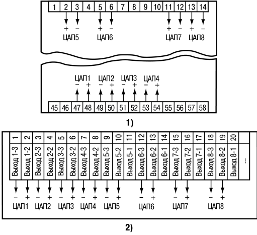
Рисунок 19 – Схема подключения твердотельных реле прибора: 1) в корпусе Щ4, 2) в корпусе Щ7
