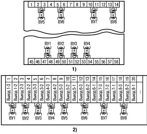
Рисунок 17 – Схема подключения симисторных оптопар прибора: 1) в корпусе Щ4, 2) в корпусе Щ7
