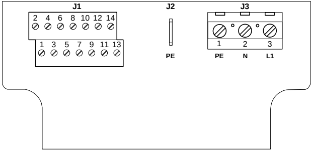
Рис. 6 Подключение клемм
