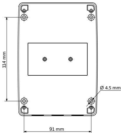
Рис. 2 Настенный монтаж интерфейсного блока
