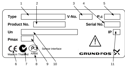
Рис. 1 Пример заводской таблички
