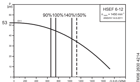
Рис. 50 Рабочий диапазон
