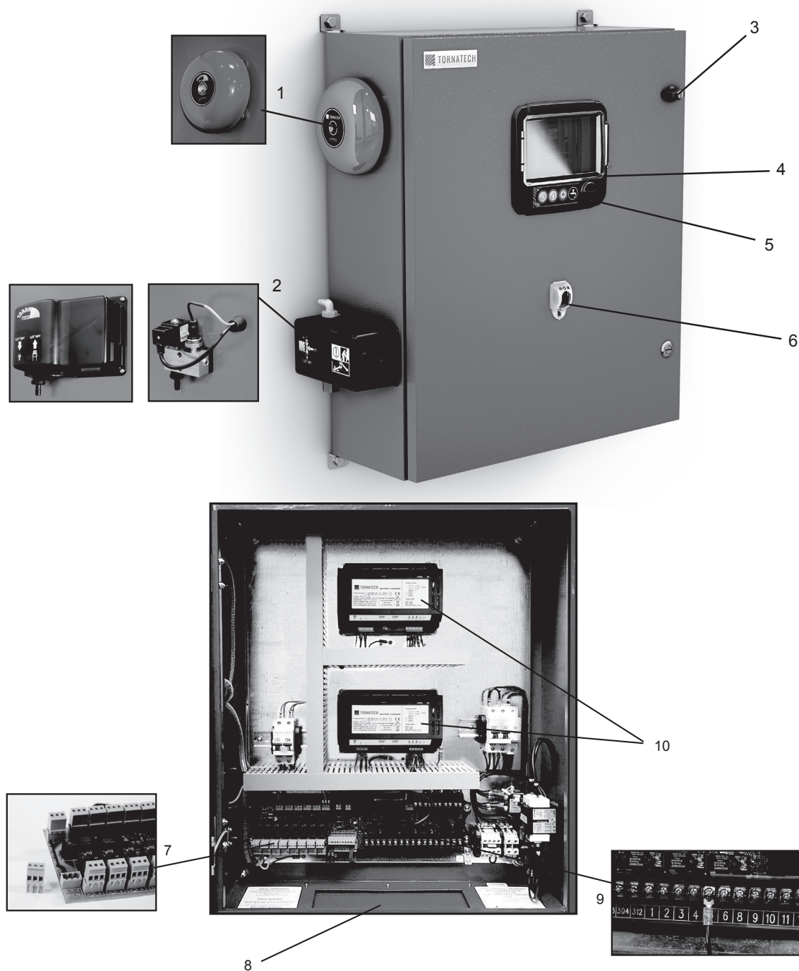
Рис. 60 Шкаф управления
