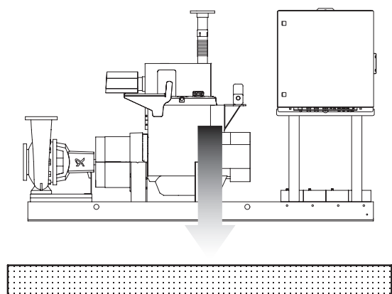
Рис. 38 Правильное расположение
