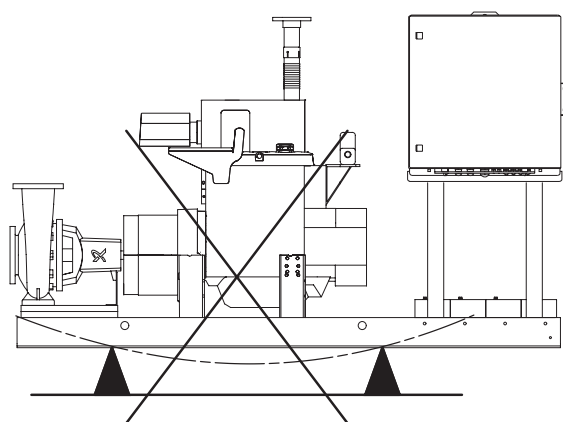
Рис. 39 Неправильное расположение
