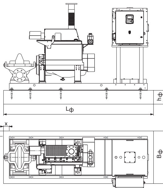
Рис. 64 Размеры основания
