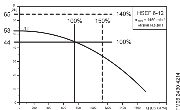
Рис. 47 Пример, зависимость давления от подачи
