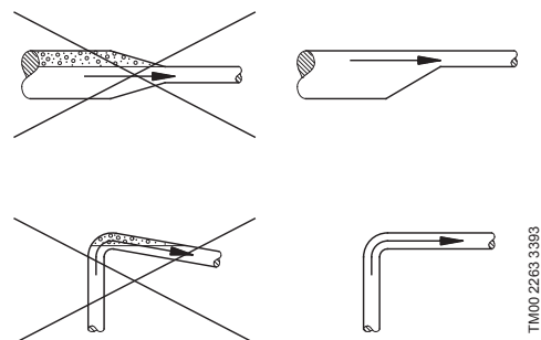
Рис. 40 Установка трубопроводов
