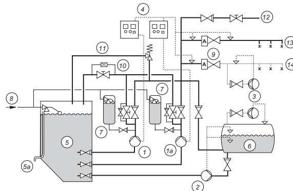
Рис. 14 Общий вид системы пожаротушения с применением установок Fire NKF
