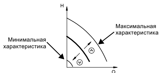
Рис. 18 Режим работы с постоянной характеристикой
