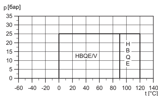
Рис. 20 Рабочий диапазон торцевых уплотнений, мощность 55 и 75 кВт
