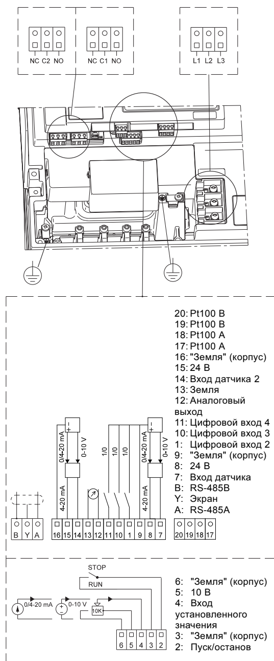
Рис. 6 Клеммы соединений, расширенный модуль ввода/вывода
