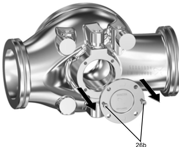
Рис. 13 Снятие фланца
