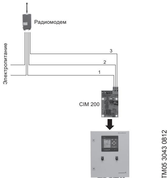
Рис. 16 Подключение радиомодема через Modbus RTU
