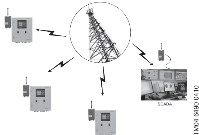
Рис. 15 Сеть радиомодема
