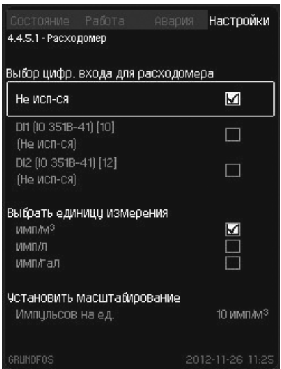
Рис. 29 Расходомер
