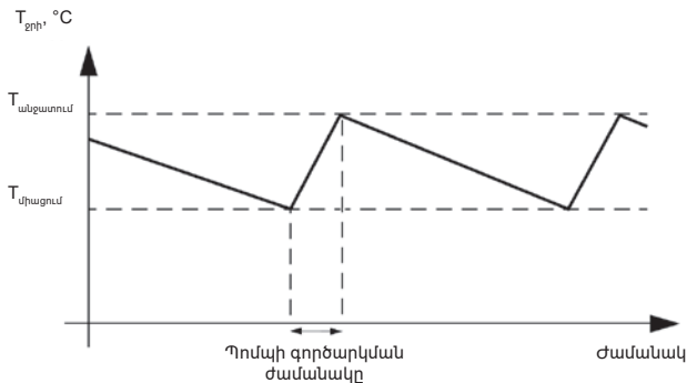
Նկար 2 Զերմաստիճանի կառավարման ռեժիմի աշխատանքի պատկերազարդումը
