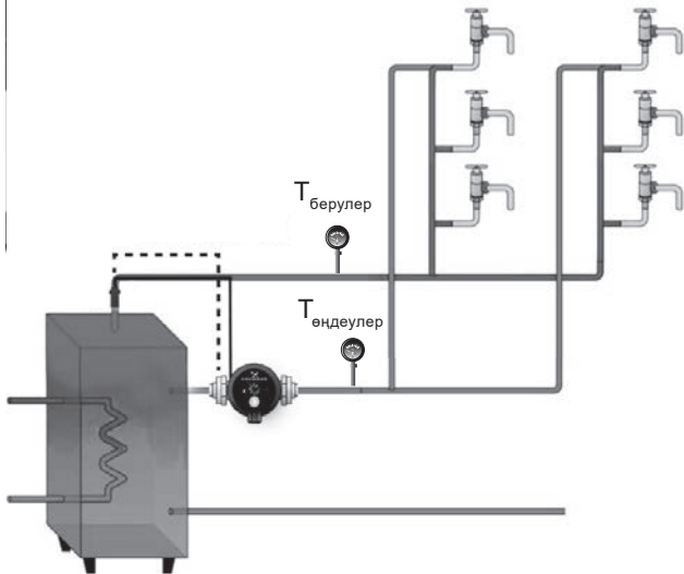
3-сур. Екі температура датчигімен ЫЖЖ жүйесіндегі COMFORT сорғысы
