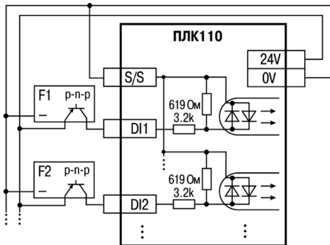
Рисунок В.3 – Подключение к дискретным входам датчиков (F1–Fn), имеющих на выходе транзисторный ключ p-n-p-типа
