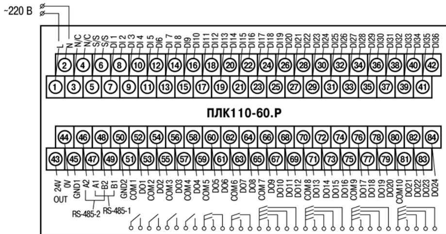
Рисунок Б.1 – Схема расположения и назначение клемм на ПЛК110-220.60.Р. Схема для ПЛК110-24.60.Р– аналогична, полярность при подключении клемм питания аналогична рисунку Б.2
