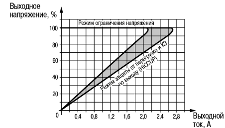
Рисунок 3 – График зависимости выходного напряжения от выходного тока (НИСОР)
