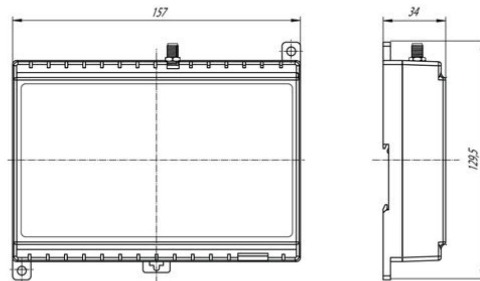
Рисунок А.1 – Габаритные размеры ПЛК323.ТЛ
