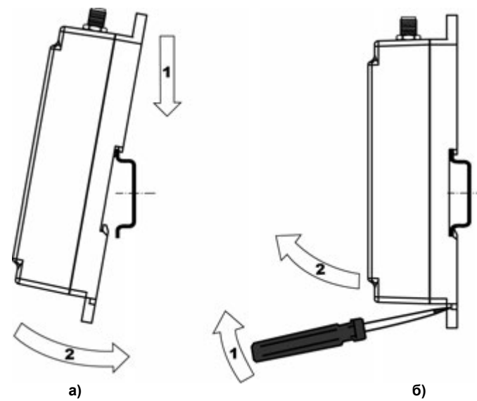
Рисунок 6.1 – Монтаж контроллера с креплением на DIN-рейку
