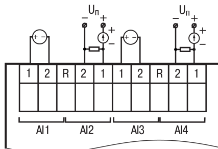
Рисунок 5.7 – Подключение датчиков с выходом в виде напряжения (к AI1 и AI3) и с выходом в виде тока (к AI2 и AI4)
