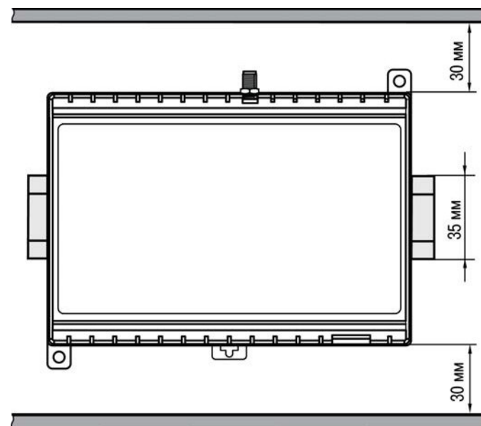
Рисунок А.3 – Расстояние до стенок корпуса КСOD при монтаже в шкаф для обеспечения вентиляции
