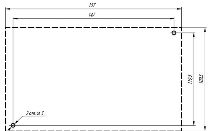
Рисунок А.2 – Разметка для установки на щит
