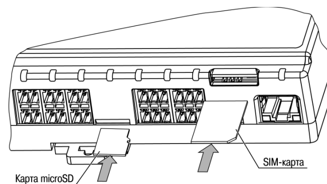
Рисунок 6.3 – Установка microSD и SIM-карты
