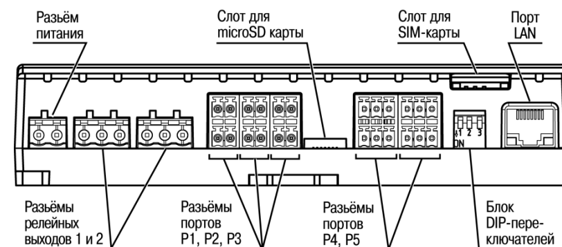
Рисунок 3.3 – Вид на нижнюю поверхность КСОД
