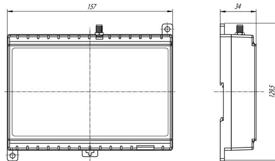
Рисунок А.1 – Габаритные размеры КСОД
