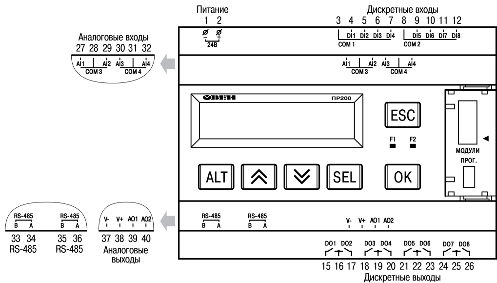
Рисунок А.14 – Расположение контактов ПР200-24.4.2.X
