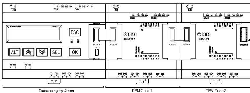
Рисунок 5.15 – Расположение модулей расширения на шине
