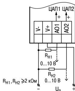
Рисунок 5.13 – Схема подключения нагрузки к ВЭ типа «У»
