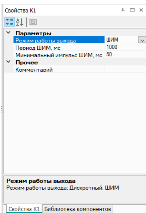
Рисунок 6.7 – Настройка параметров работы выхода типа К в режиме ШИМ
