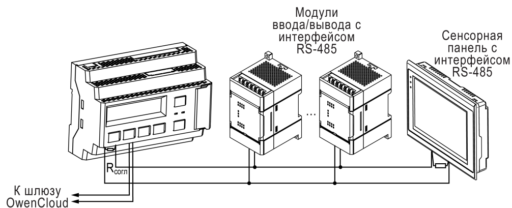
Рисунок 5.18 – Смешанная схема подключения
