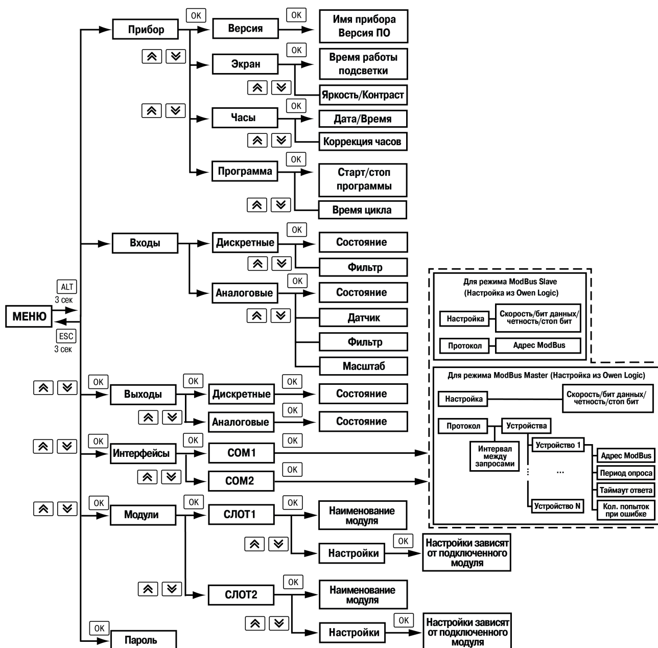
Рисунок 7.2 – Структура системного меню
