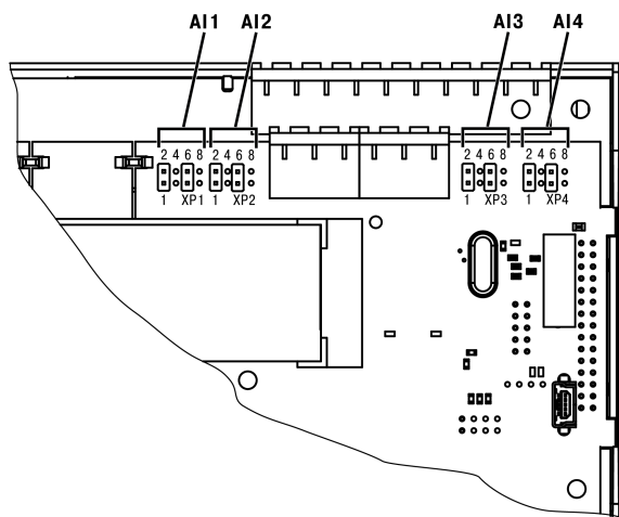
Рисунок 6.3 – Схема расположения перемычек
