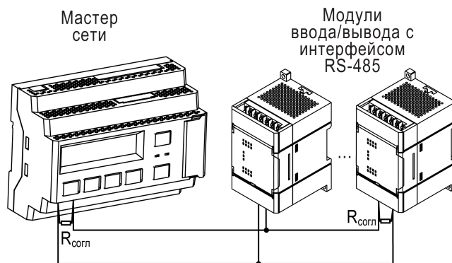
Рисунок 5.17 – Типовая схема подключения для ПР200 в режиме Master
