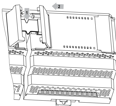
Рисунок 5.14 – Укладка шлейфа в углубление
