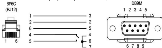
Рисунок В.2 - Схема кабеля KC3 для подключения модема к ПЛК150 по интерфейсу RS-232
