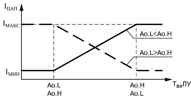
Рисунок 7.9 – Выходные характеристики ЦАП
