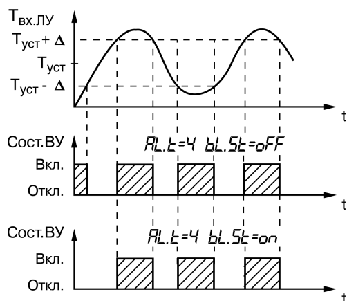
Рисунок 7.6 – Диаграммы работы ЛУ при различных значениях параметра bL.St
