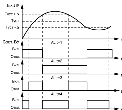
Рисунок 7.5 – Выходные характеристики компараторов
