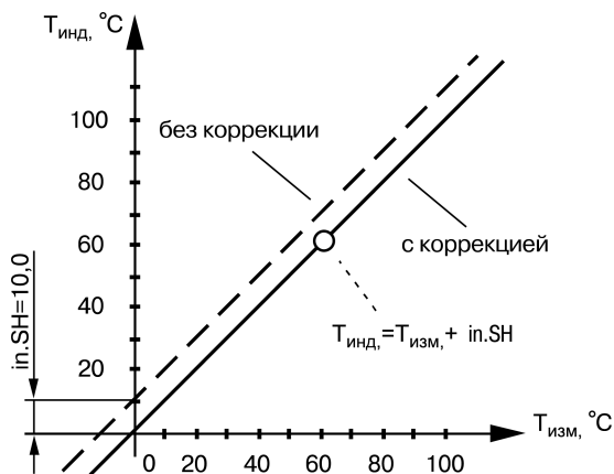
Рисунок 7.3 – Коррекция «сдвиг характеристики»
