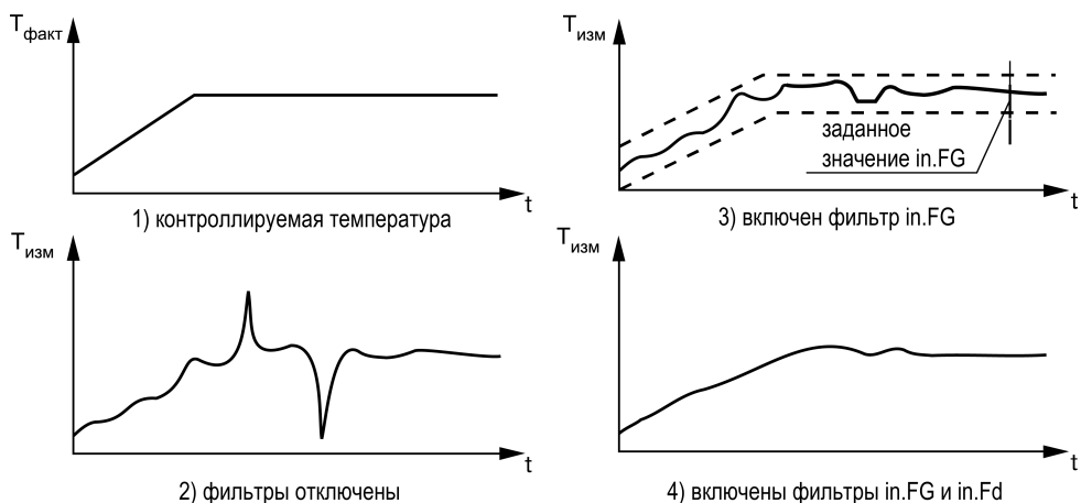
Рисунок 7.2 – Временные диаграммы работы цифровых фильтров
