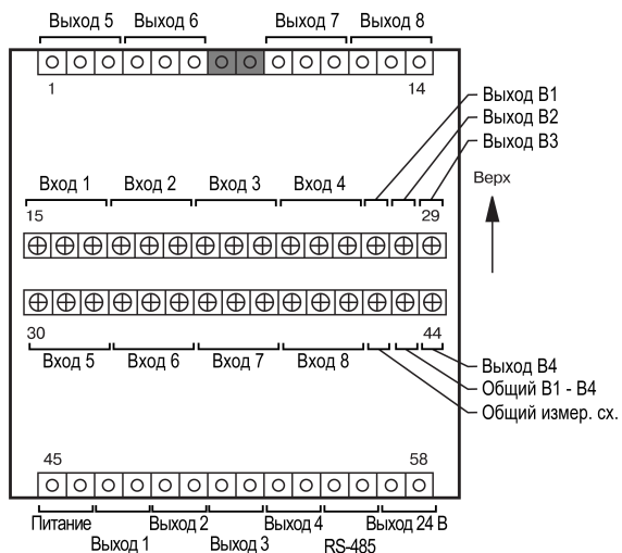
Рисунок 5.2 – Клеммник TPM138В
