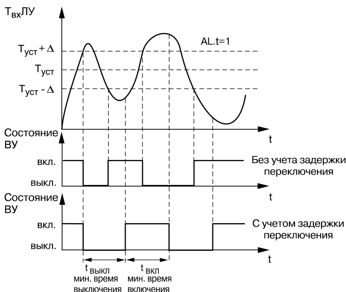
Рисунок 7.8 – Работа ЛУ с заданным временем удержания
