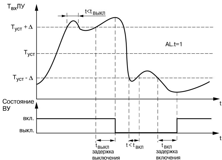
Рисунок 7.7 – Работа ЛУ с задержками включения и выключения
