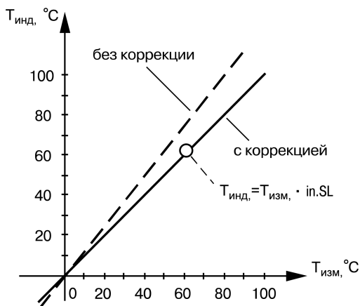
Рисунок 7.4 – Коррекция «наклон характеристики»
