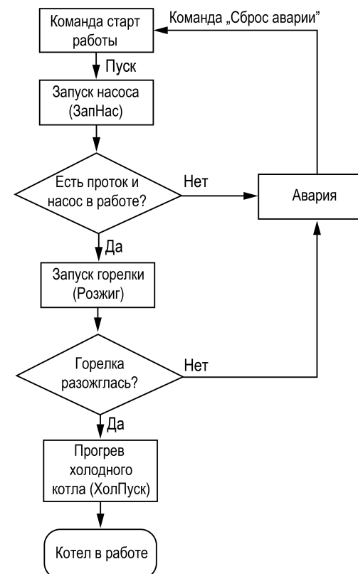
Рисунок 9.1 – Алгоритм запуска
