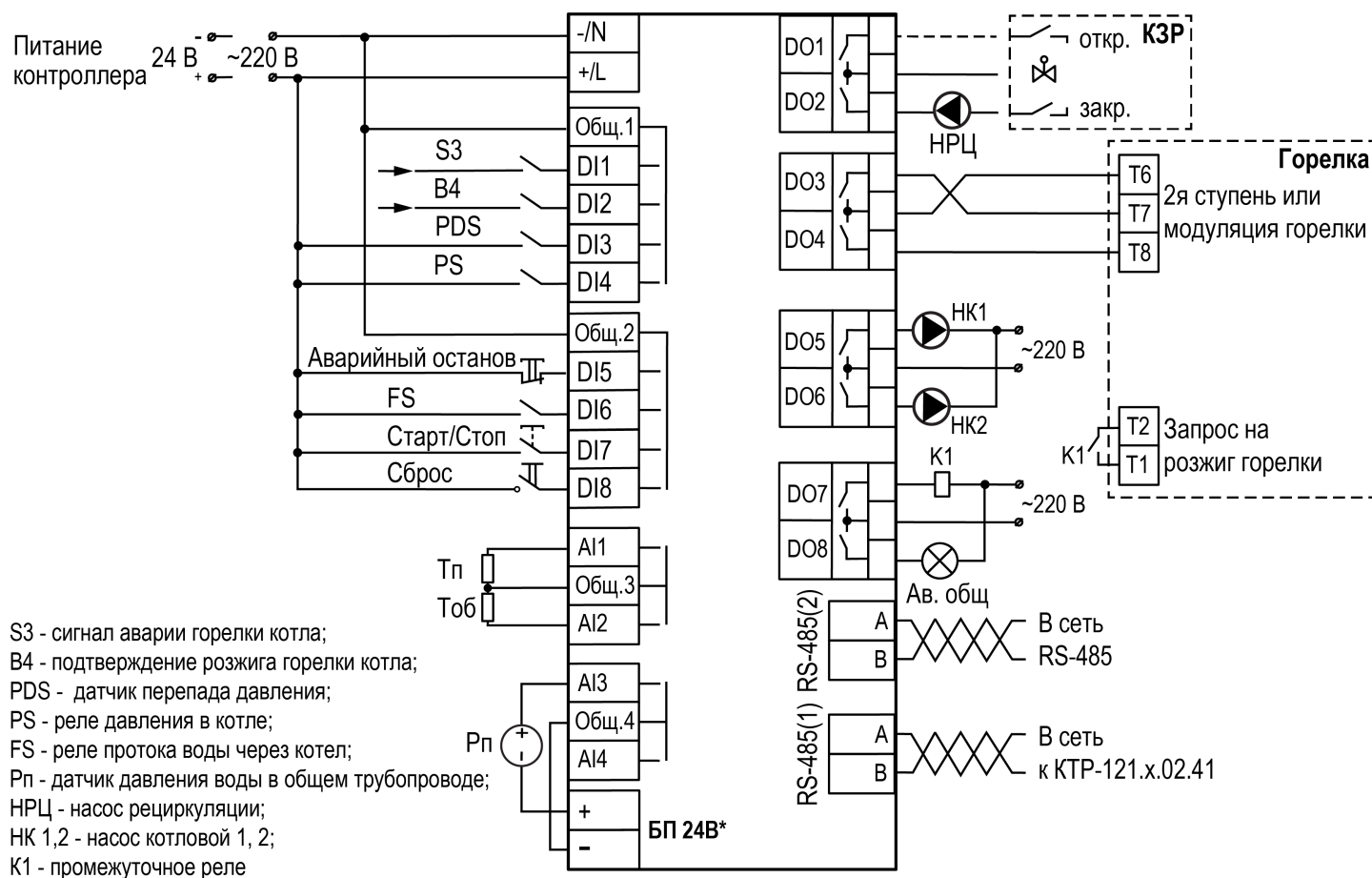
Рисунок 6.4 – Схема подключения
