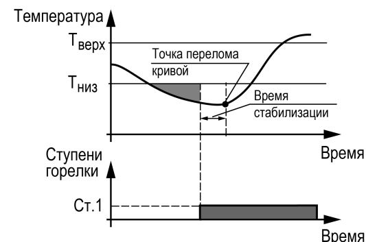
Рисунок 9.3 – Принцип определения Вр.Стаб
