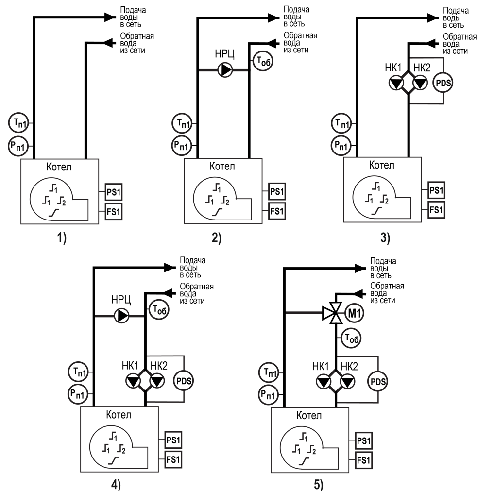
Рисунок 1.1 – Объект управления
