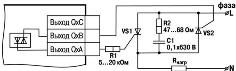
Рисунок 6.4 - Схема подключения к ВУ типа С двух тириستоров, подключенных встречно-параллельно
