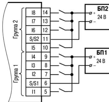
Рисунок 6.10 – Схема подключения к ПР114 дискретных датчиков с выходом типа «сухой контакт»
