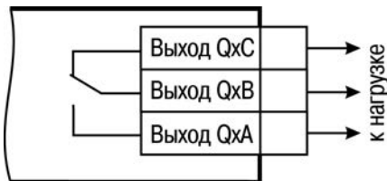
Рисунок 6.1 - Схема подключения нагрузки к ВЭ типа Р
