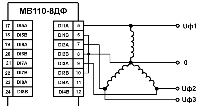
Рисунок Б.4 - Схема подключения к МВ110-8ДФ трехфазного двигателя (пример контроля обрыва питающих фаз)
