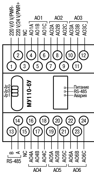
Рисунок Б.1 - Общий чертеж МУ110-6У
