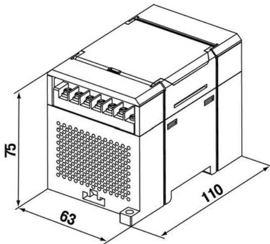
Рисунок А.1 – Габаритный чертеж МВ110-224.1ТД
