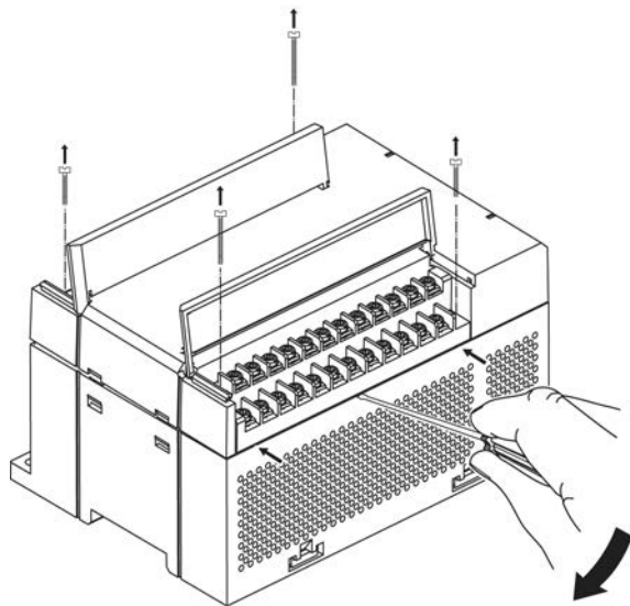
Рисунок Д.2 – Отделение клеммной колодки от прибора MB110-224.4ТД
