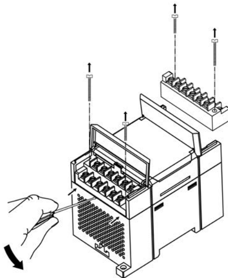
Рисунок Д.1 – Отделение клеммной колодки от прибора MB110-224.1ТД
