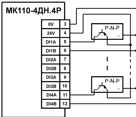
Рисунок Б.5 – Схема подключения к МК110-220.4ДН.4Р дискретных датчиков с транзисторным выходом р-n-p-типа
