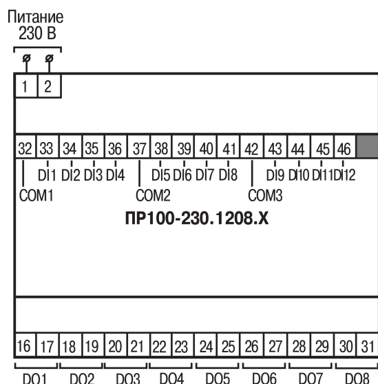
Рисунок 5.5 – Расположение контактов для PR100–230.1208.x
