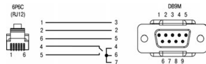
Рисунок В.2 - Схема кабеля КС3 для подключения модема к ПЛК100.ТЛ по интерфейсу RS-232
