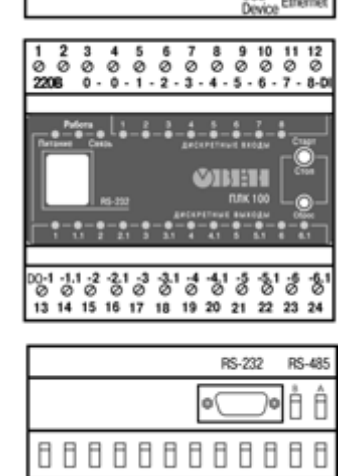
Рисунок 5.1 - Внешний вид) и ПЛК100-220.ТЛ
