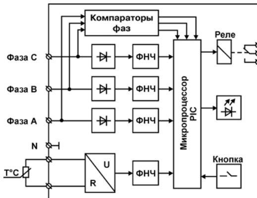
Рисунок 3.2 – Функциональная схема МНС1
