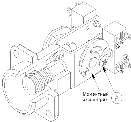
Рис.3 Ограничитель крутящего момента
